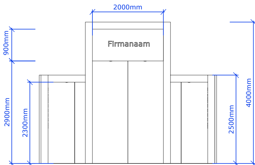
Vooraanzicht
