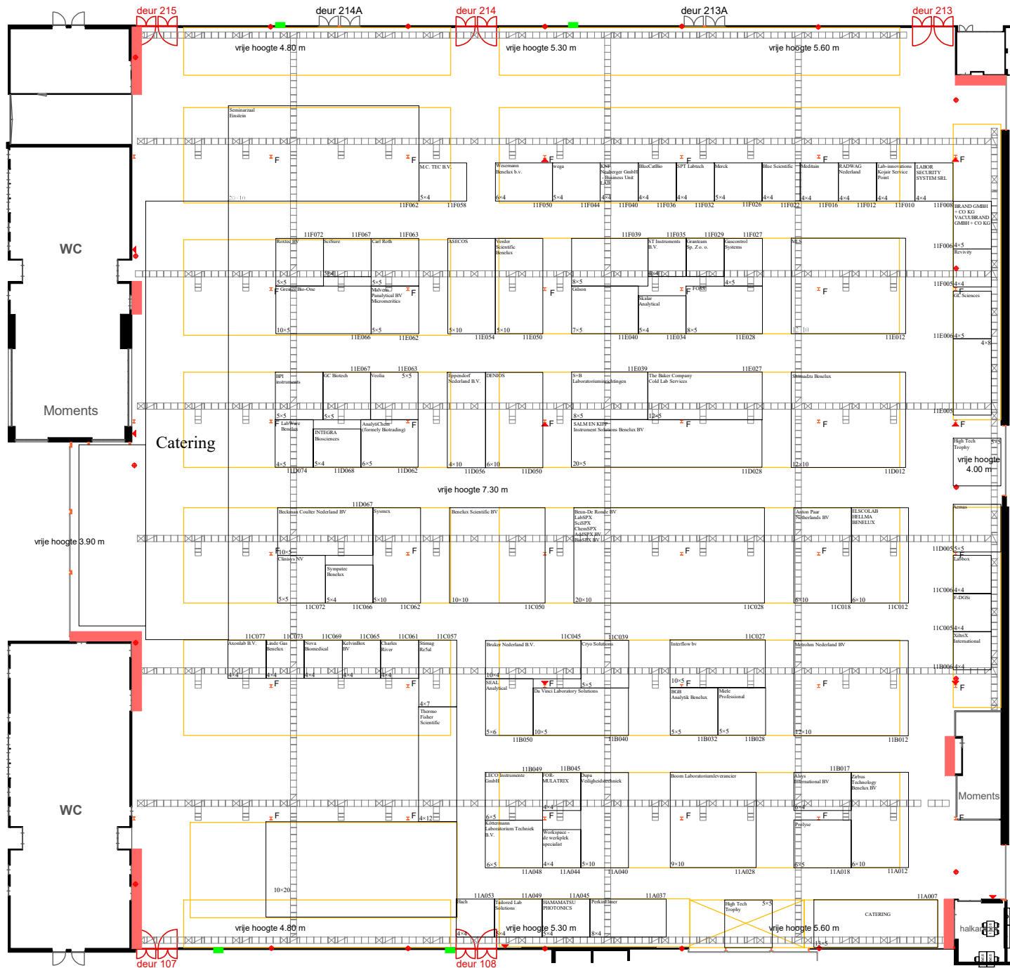
Hal 11 vrije hoogte hal 7.30 m
